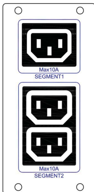
Σχήμα 22: Τμηματοποίηση φορτίων
