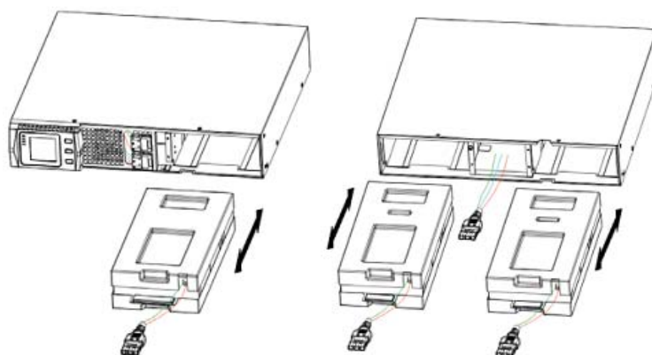
Σχήμα 24 Αφαίρεση ερμαρίου συσσωρευτών
