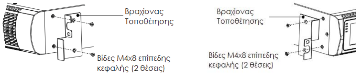
Σχήμα 5 Τοποθέτηση των βραχιόνων
